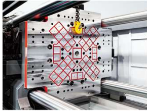
Mag Clamp MGA
